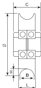
Doble rodamiento Double bearing Double roulement
