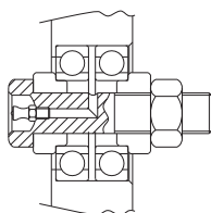
Eje engrasador Axix with greaser Axe graisseur
